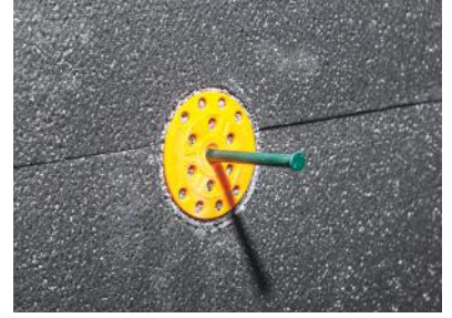
Şekil 3 Açılan dübel deliğine dübeller yerleştirilerek dübel çivileri tamamen çakılır.
